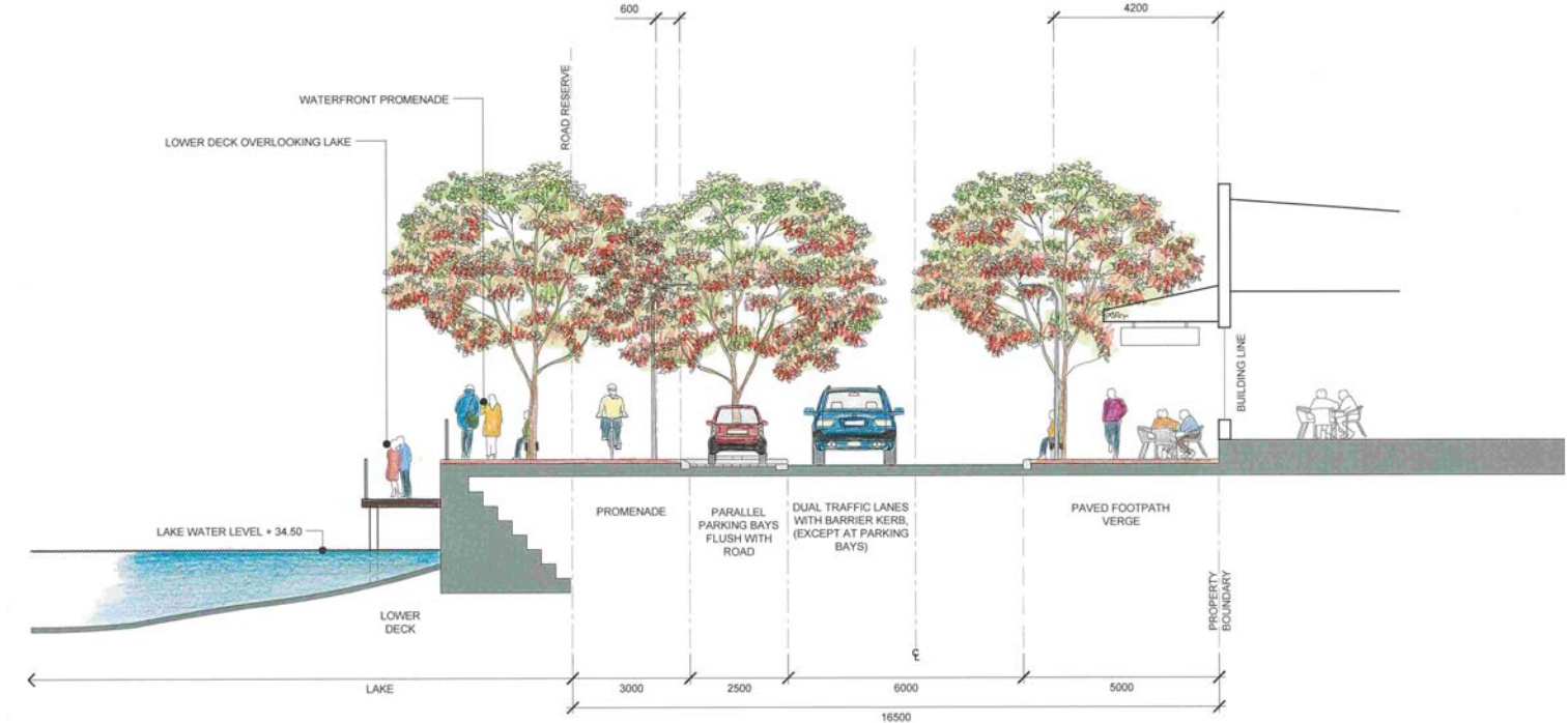
B SECTION B : PROMENADE 1:100 @ A3
